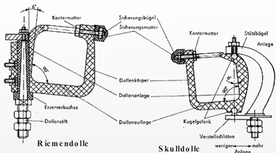
Dollen (Halterung für Ruderblätter) im Detail
